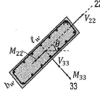
Şekil E.1 Perde İç Kuvvetleri
