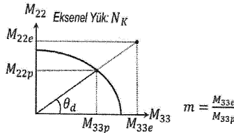
Şekil D.2 M_{22} - M_{33} Etkileşim Diyagramı
