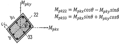
b) Kirişlerin mafsallaşması ile oluşan kolon momentleri
