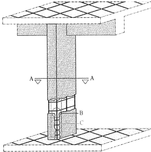
Şekil B.1 Kolon Beton Pas Payı Sıyırma Örneği
