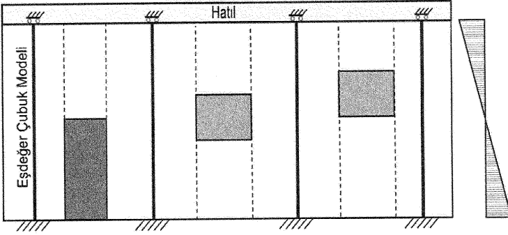
a) Eşdeğer Çubuk Modeli
