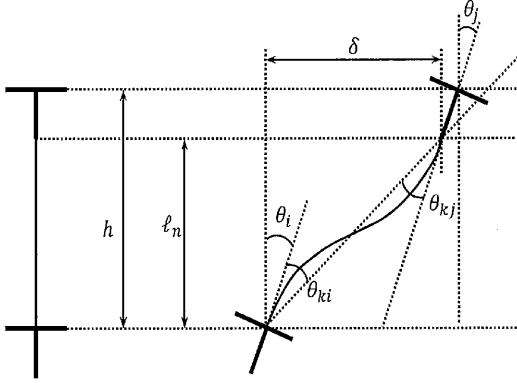
Şekil G.1 Eleman Yer Değiştirme Eksen Dönmesi Hesabı
