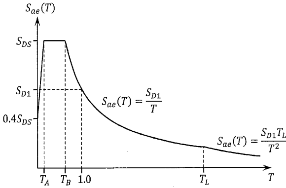
Şekil 2.1 Yatay Elastik İvme Spektrumu
