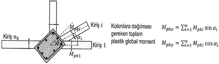
a) Kolon-kiriş birleşim bölgesi
