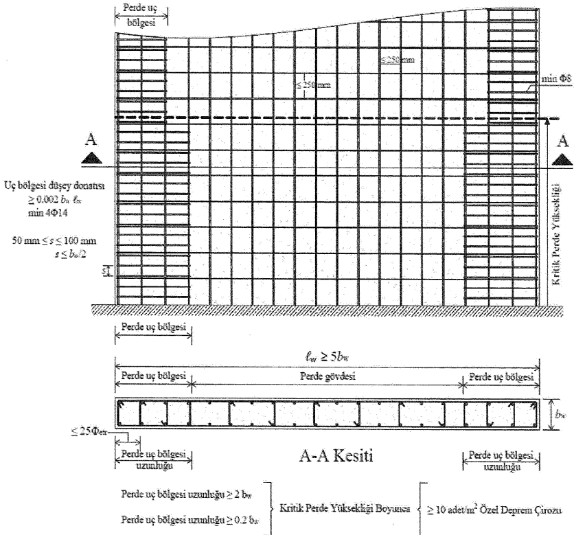
Şekil E.2 Perde Başlık Bölgesi
