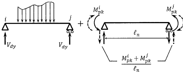
Şekil D.5 Kiriş Kesme Kuvveti
